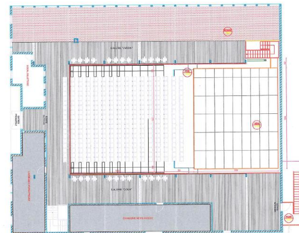
PLAN GALERIE - ECH: 1/100 - Configuration 2 (fosse haute + scène longue)
