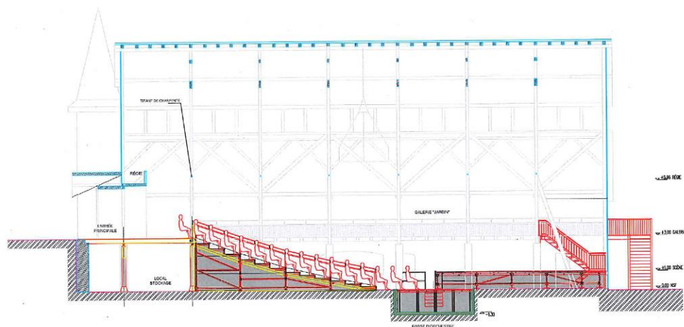
COUPE LONGITUDINALE - ECH: 1/100 - Configuration 2 (fosse haute + scène longue)
