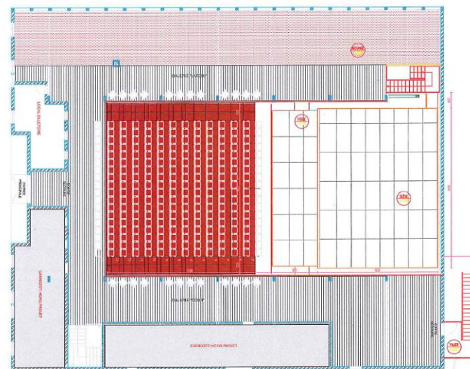
PLAN GALERIE - ECH: 1/100 - Configuration 1 (fosse basse + scène en porte à faux)
