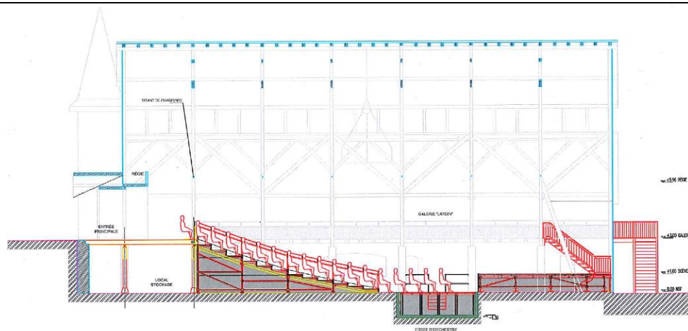
COUPE LONGITUDINALE - ECH: 1/100 - Configuration 3 (fosse haute + scène courte)
