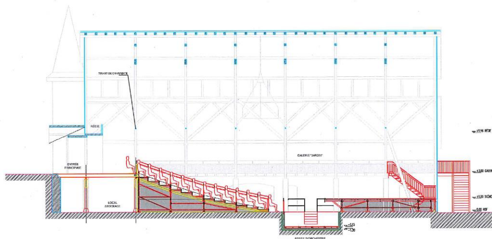
COUPE LONGITUDINALE - ECH: 1/100 - Configuration 1 (fosse basse + scène en porte à faux)
