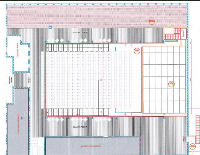
PLAN GALERIE - ECH: 1/100 - Configuration 3 (fosse haute + scène courte)
