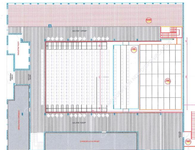
PLAN GALERIE - ECH: 1/100 - Configuration 4 (gradinage fosse + scène courte basse)
