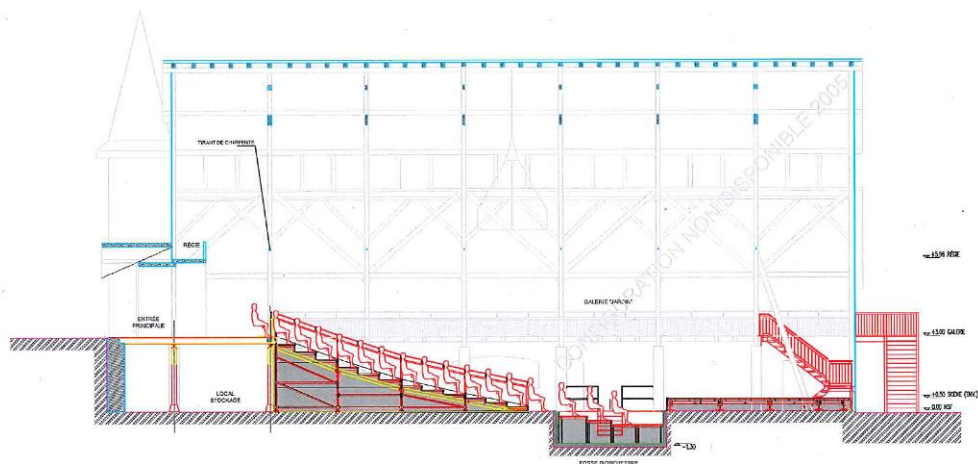
COUPE LONGITUDINALE - ECH: 1/100 - Configuration 4 (gradinage fosse + scène courte basse)
